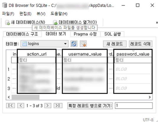
(그림 2) Login Data.sqlite에 저장된 사용자 로그인 정보
